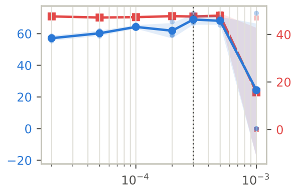
MiLoRA
