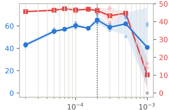
MiLoRA
