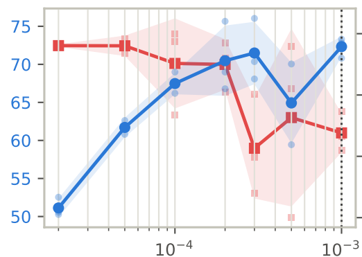
LoRA-Null
